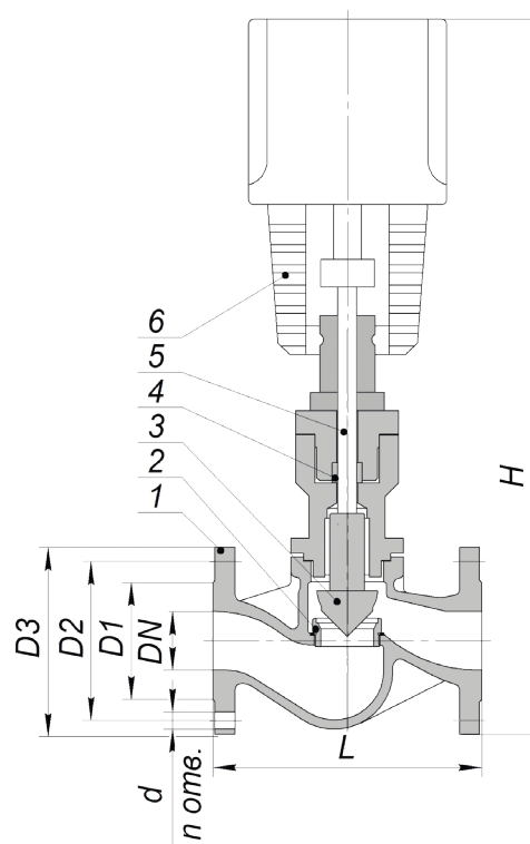
Клапан на пар с приводом ТНК
