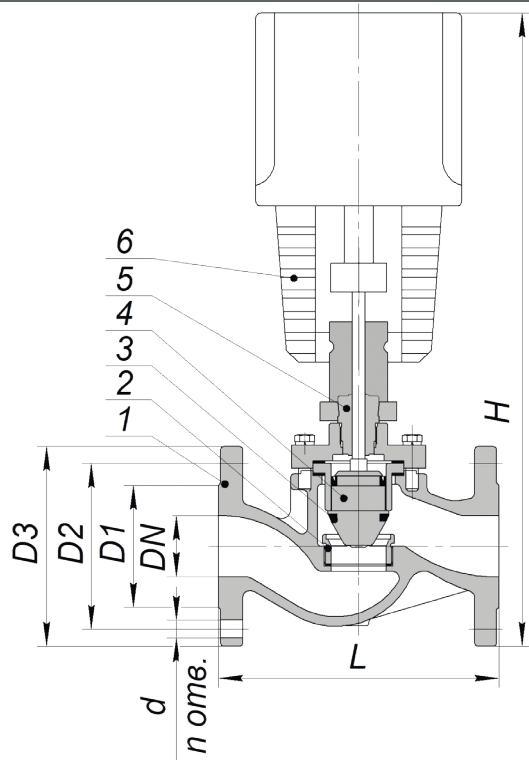
Клапан с приводом ТНК
